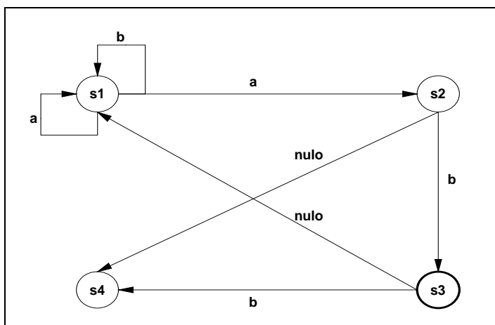
Figura 7.3 Um autômato finito não determinístico
